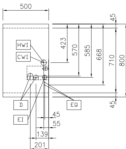
Boven aanzicht
